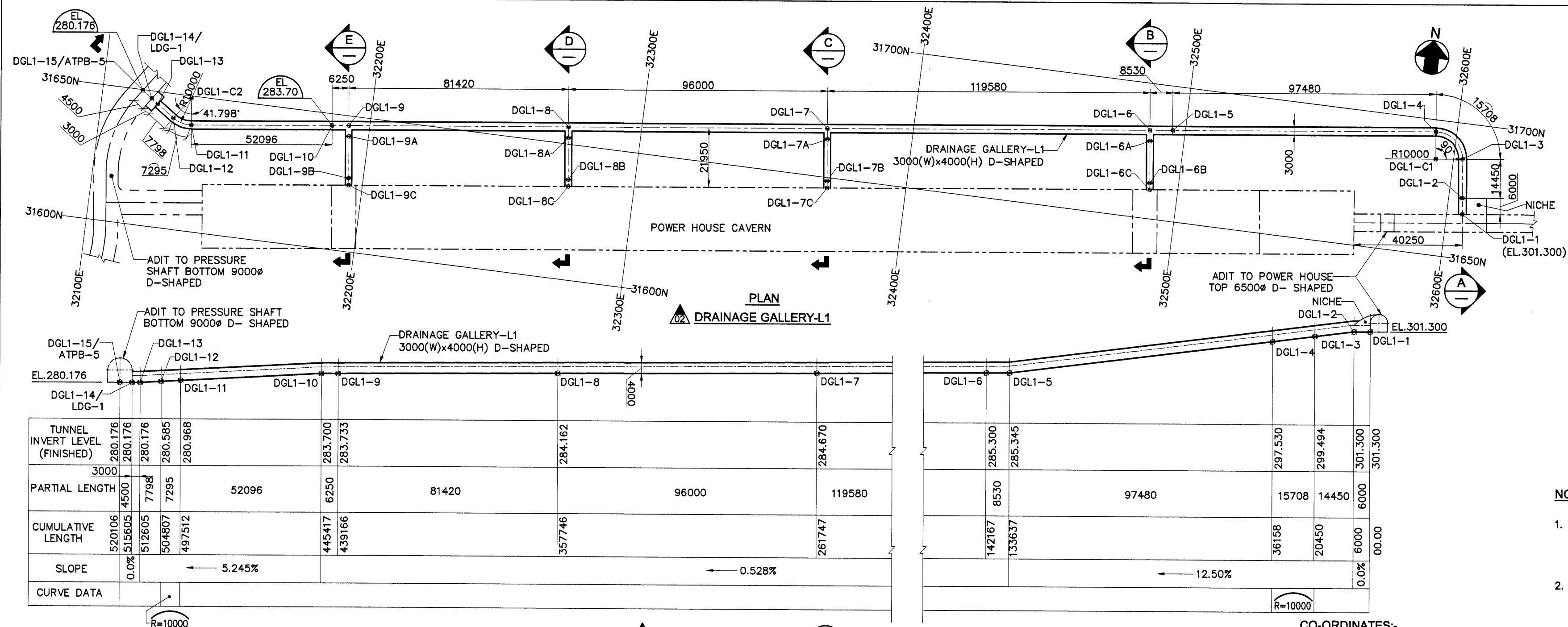
LONGITUDINAL SECTION (A)
