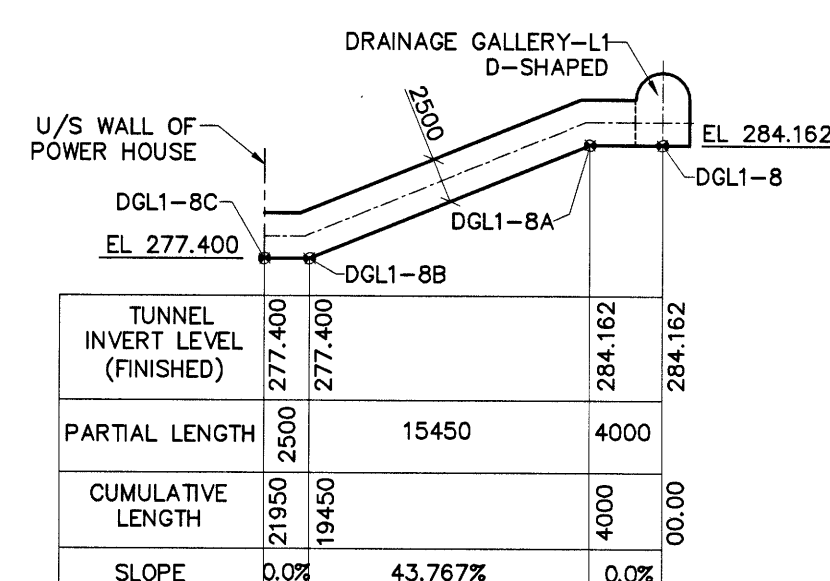
SECTION D (NTS)
